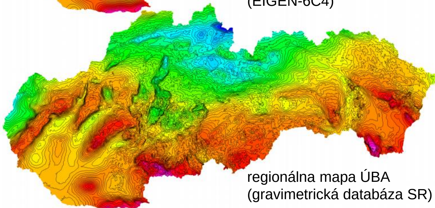
mapa ÚBA z GGM modelu (EIGEN-6C4)
