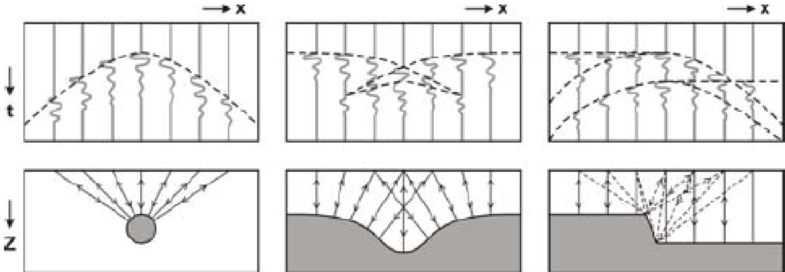
príklady – izolovaný objekt, (jedna difrag. vlna)
