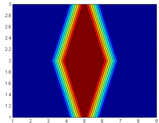
riešenie podľa Last and Kubik (1983), 10. iterácia
