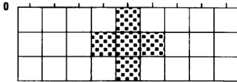
riešenie podľa Last and Kubik (1983), 2. iterácia
