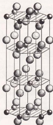
Fig. 61. \text{CdCl}_2 -Gitter (aus EASST).
