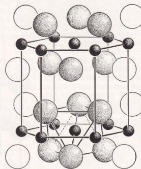
Fig. 62. \text{CdI}_2 -Gitter (aus EASST).
